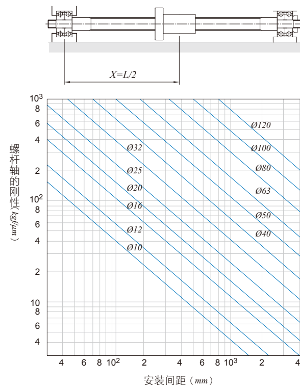
图18. 丝杠轴刚性图表(固定-固定)
