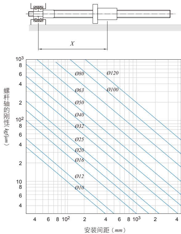
图17. 丝杠轴刚性图表(固定-自由)
