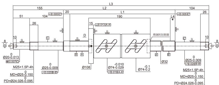
滚珠丝杠规格
