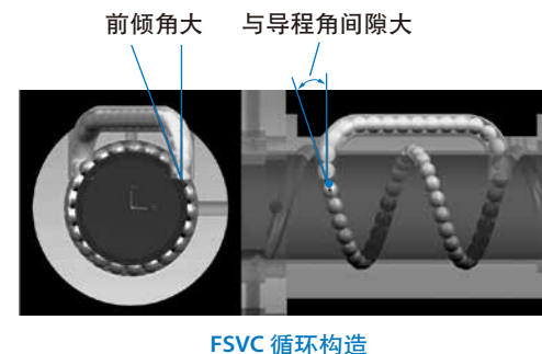
图6. 旧型式 FSVC 循环构造
