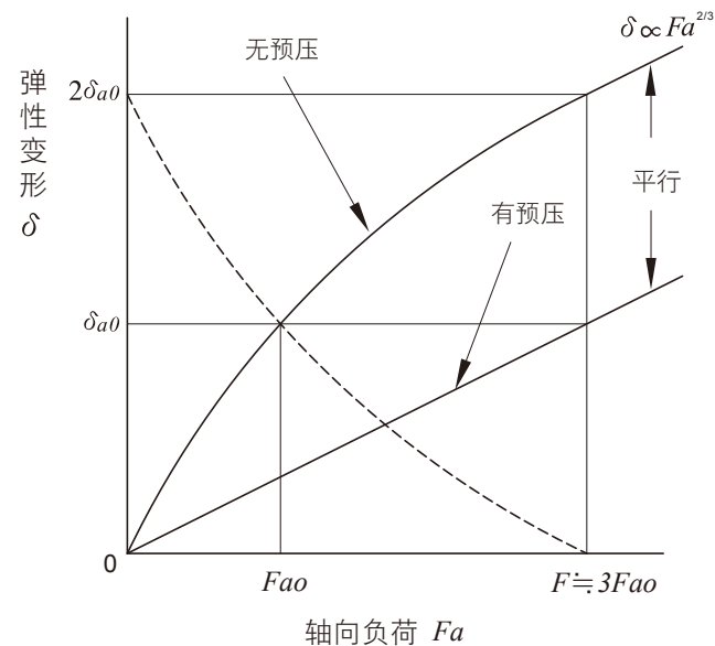
图25. 弹性变形曲线
