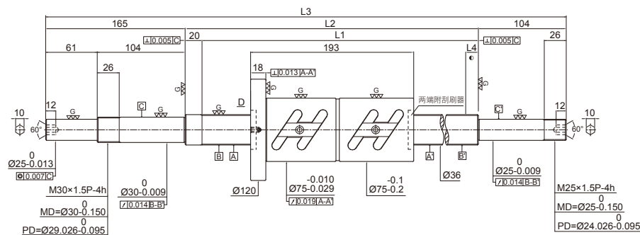
滚珠丝杠规格
