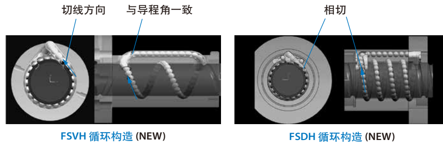
图5. FSVH、FSDH循环构造
