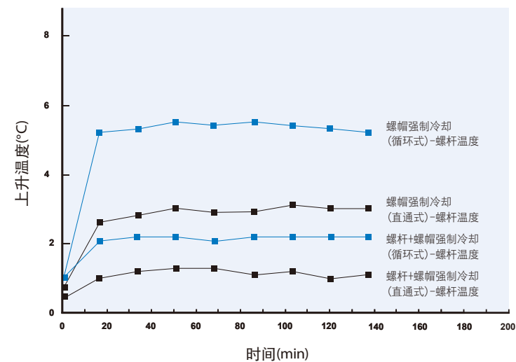
图46. 循环式与直通式比较
