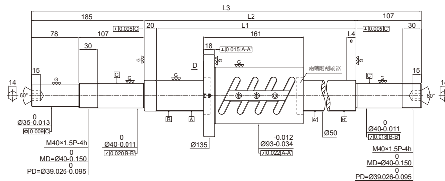
滚珠丝杠规格
