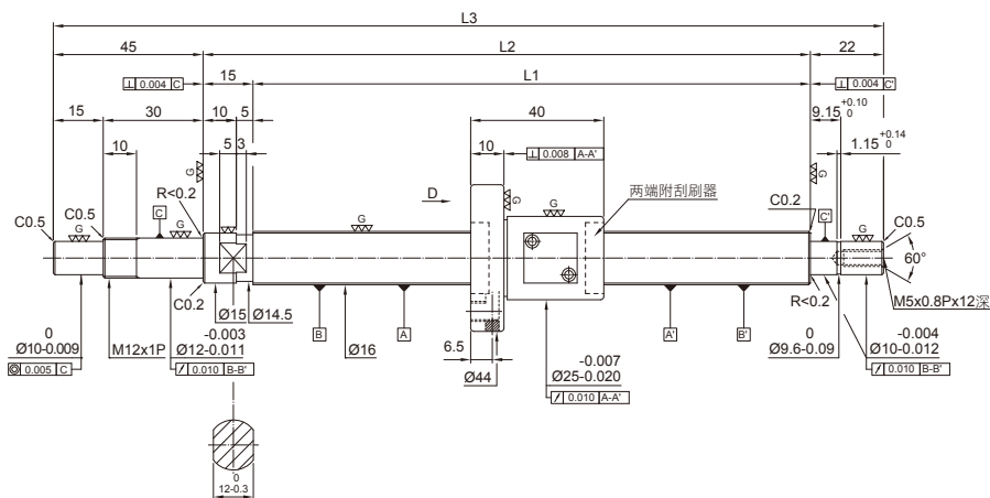
滚珠丝杠规格
