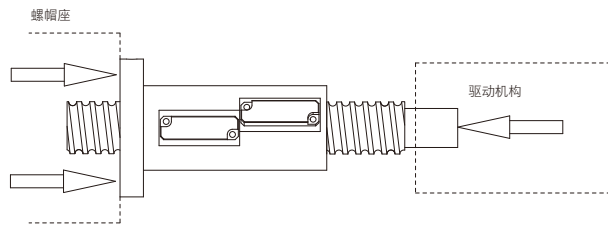
图7. 高负荷丝杠建议安装方式
