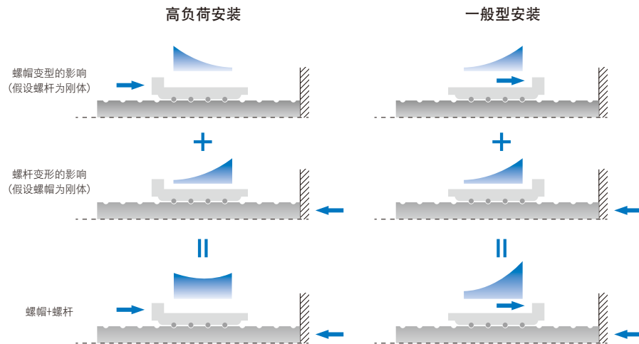
图8. 负载分布图
