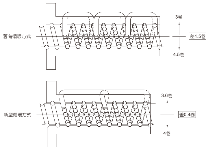
图4. 高负荷丝杠新旧循环圈数差异比较
