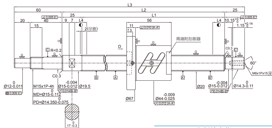
滚珠丝杠规格
