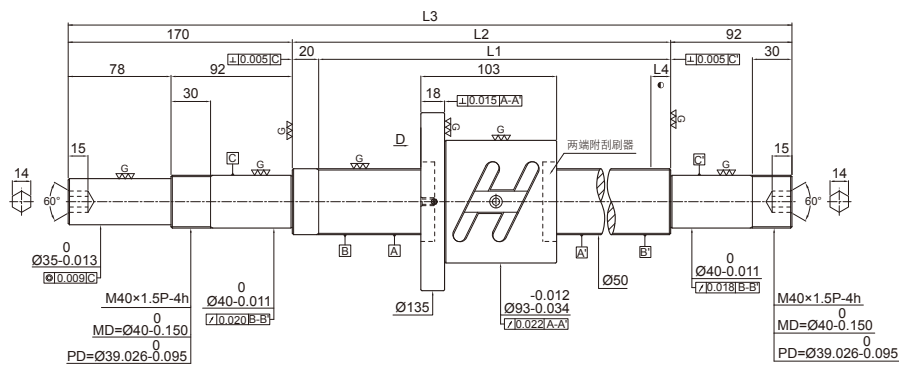
滚珠丝杠规格
