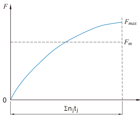
图29. 呈正弦曲线变动的负荷二
