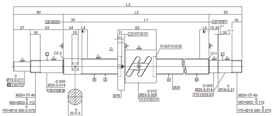
滚珠丝杠规格
