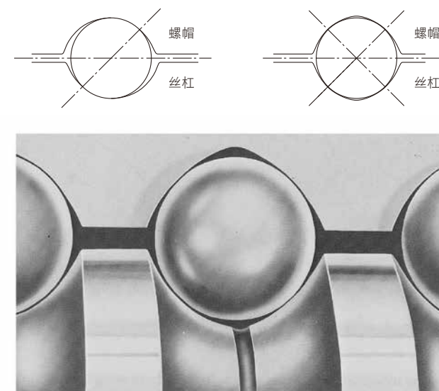
图2. 哥德式螺纹
