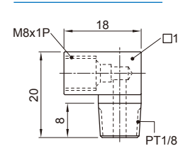
OL-D型
