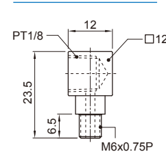
OL-A型
