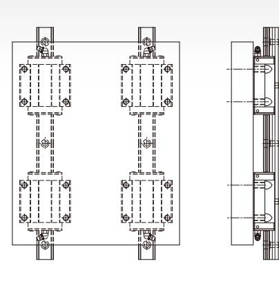
垂直方式(代码：V)
