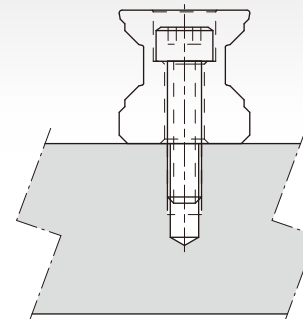
沉头孔型 (R型)
