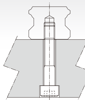
螺纹孔型 (T型)
