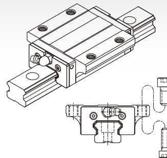
MSB-LE 型
