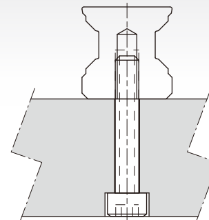
螺纹孔型 (T型)
