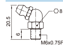
G-M6型
