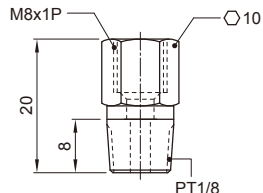
OS-D型
