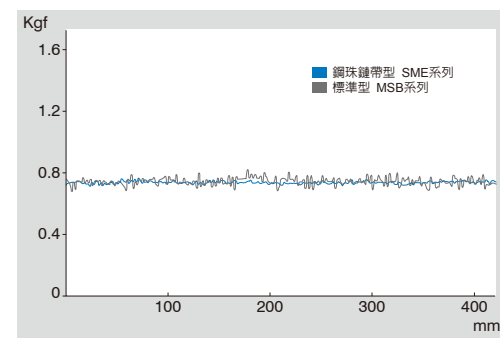
推力值比较
