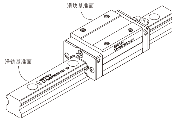
滑轨的标记
