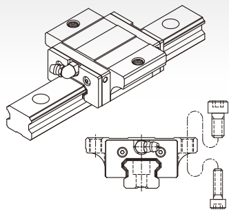
MSB-TE 型
