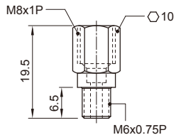
OS-D型
