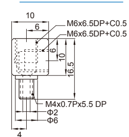
OL-C型
