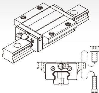
MSB-E 型
