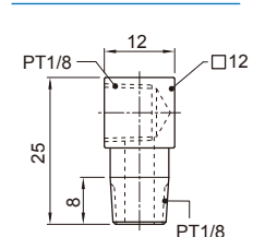
OL-C型
