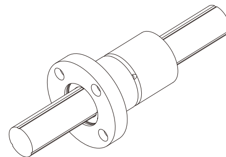
圖2. 法蘭型滾珠花鍵SLF型
