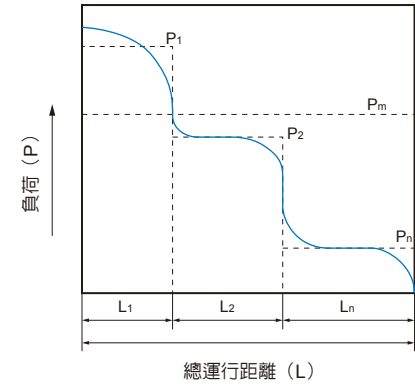
圖18. 階段變動負荷
